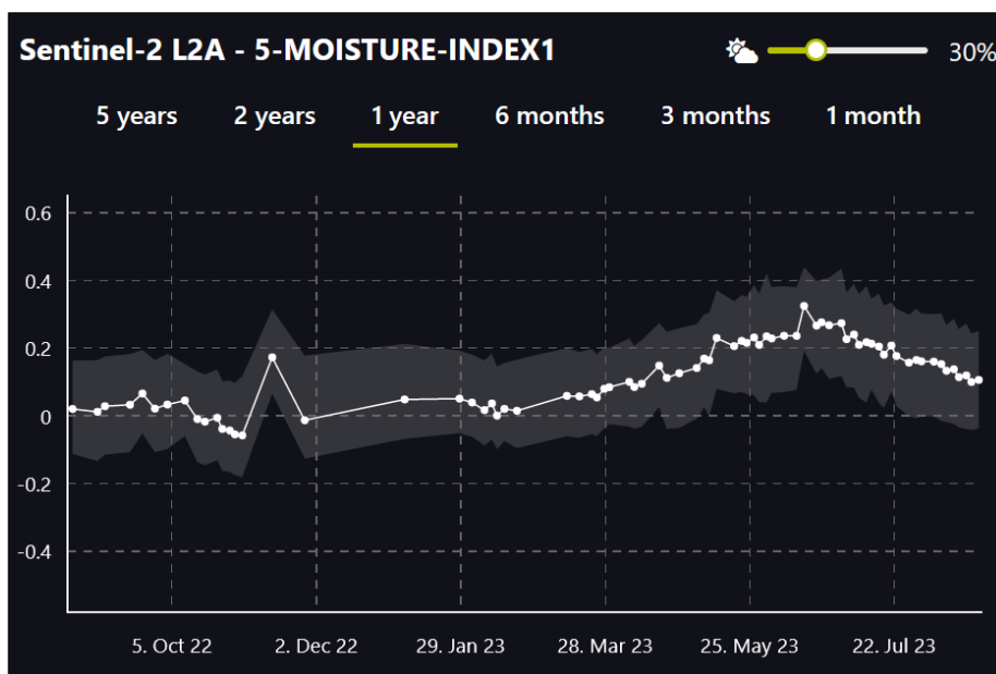
Sl. 30. Srednje vrijednosti indeksa vlažnosti tla – zapadni dio Blatskog polja (8. 2022. - 8. 2023.)
